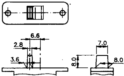
MIDDLE KNOB
