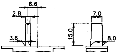
LONG KNOB
